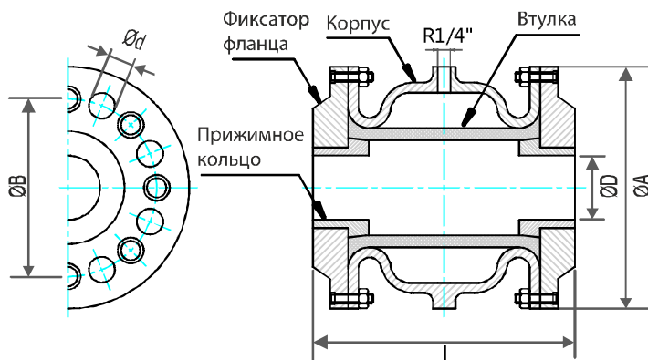
Фланцевый пережимный клапан
