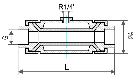
Резьбовый пережимный клапан
