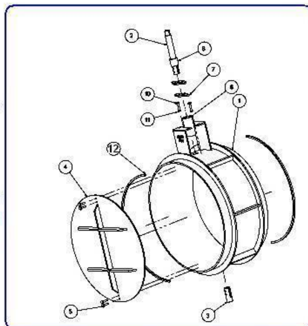
Рис.1 Конструкция заслонок НТ
